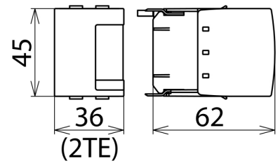
Maßbild DV MOD 255
