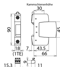
Maßbild DG S 320 FM
