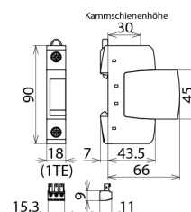
Maßbild DG S 385 FM
