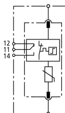
Principalschaltbild DG S 440 FM
