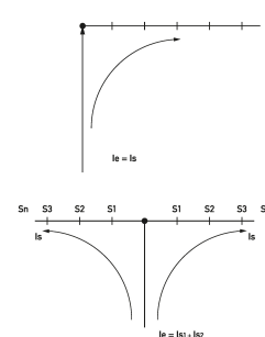
Diagramm Stromverteilung
