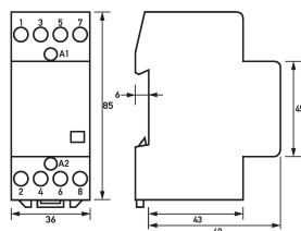
Maßzeichnung Gruppenansicht
