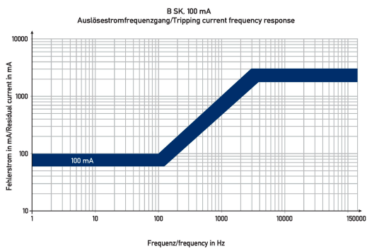
Diagramme Fehlerstromschutzschalter DFS 4 016-4/0,10-B SK
