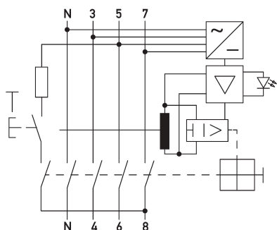
Schaltungsbeispiel Fehlerstromschutzschalter DFS 4 080-4/0,50-B SK
