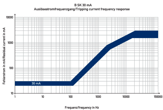
Diagramme Fehlerstromschutzschalter DFS 4 100-4/0,03-B SK
