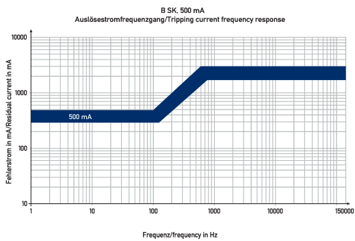
Diagramme Fehlerstromschutzschalter DFS 4 100-4/0,50-B SK
