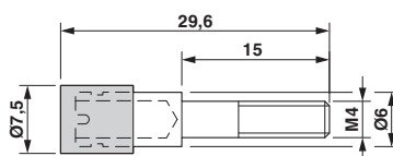
Maßzeichnung
