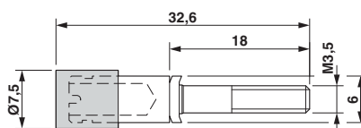
Maßzeichnung
