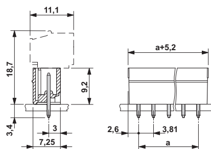
Maßzeichnung
