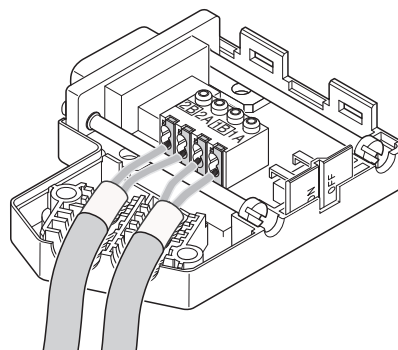
Rechtsseitige Kabelzuführung
