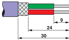
Abisolierangaben
