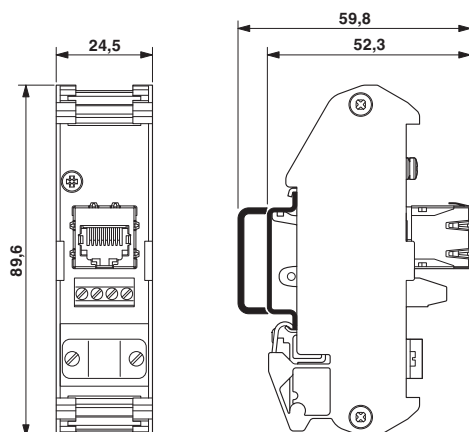
Maßzeichnung
