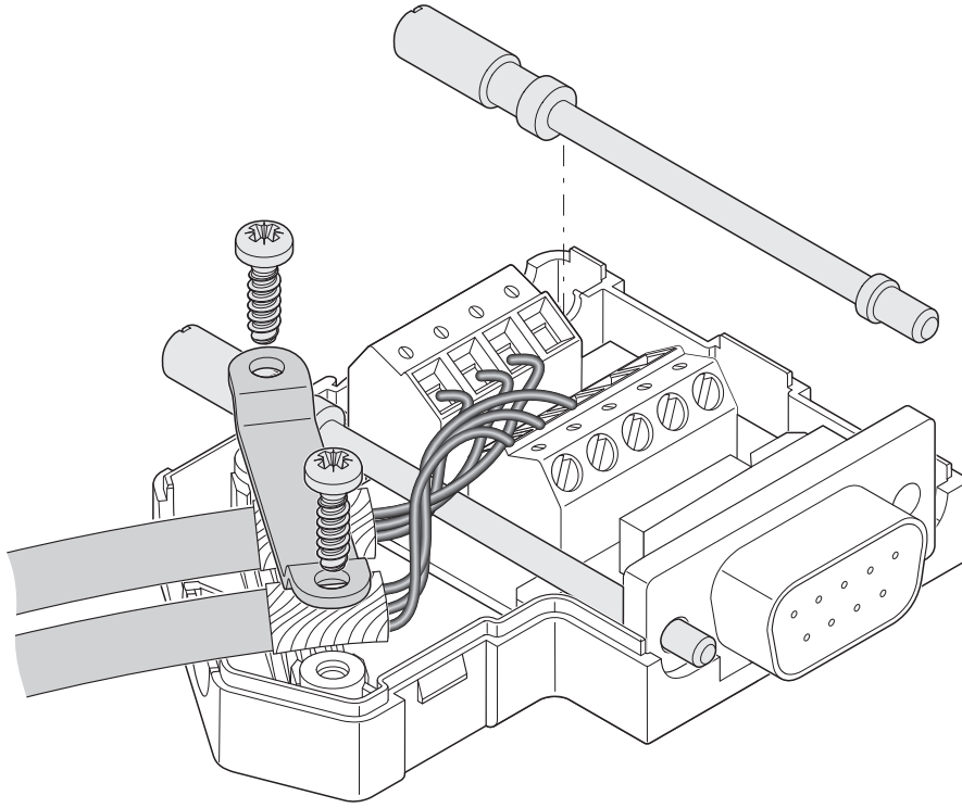
Schemazeichnung
