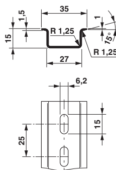
Maßzeichnung
