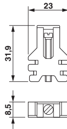
Maßzeichnung
