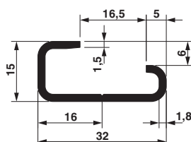
Maßzeichnung
