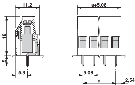
Maßzeichnung
