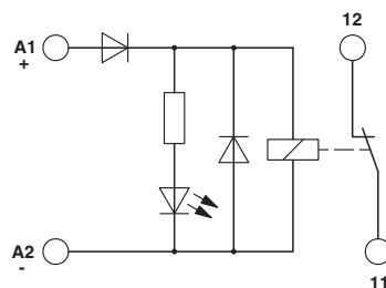
Schaltplan
