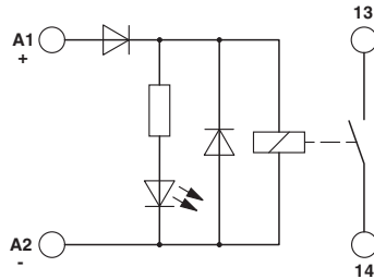
Schaltplan
