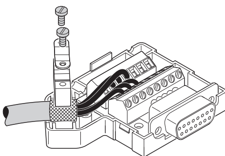
Schemazeichnung
