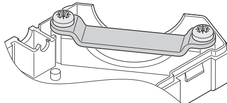
Schemazeichnung
