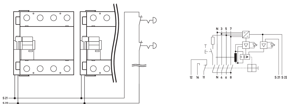
Schaltungsbeispiel Fehlerstromschutzschalter DFS 4 040-4/0,03-B SK NA
