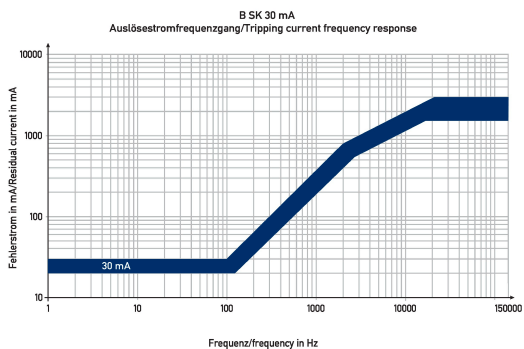
Diagramme Fehlerstromschutzschalter DFS 4 040-4/0,03-B SK NA
