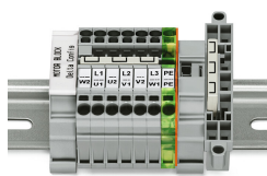
Dieser speziell für die Herstellung einer Dreieckschaltung entwickelte Dreieck-brücker findet bei Motorklemmbrettern mit Reihen-klemmen TOPJOB® S seinen Einsatz.
