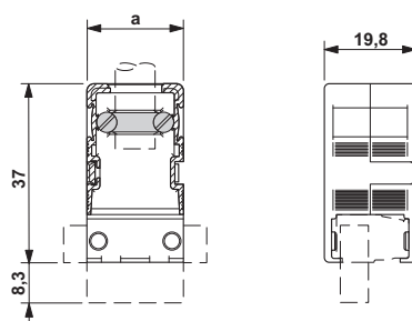
Maßzeichnung
