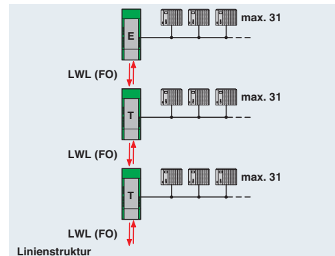
Applikationszeichnung
