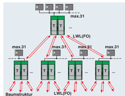
Redundante Sternstruktur
