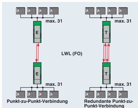
Redundante Punkt-zu-Punkt-Verbindung
