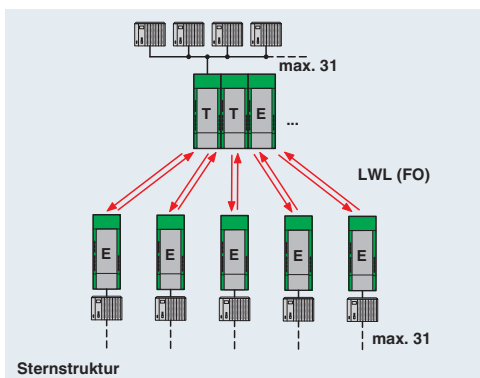
Applikationszeichnung
