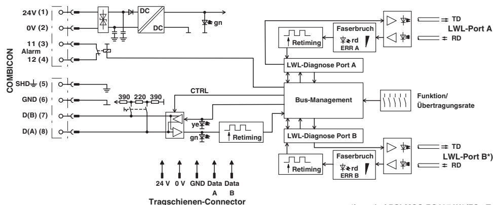
Blockschaltbild
