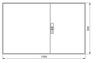
ZB15S
