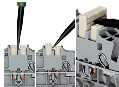
Kammbrücke lösen Mit dem Betätigungswerkzeug zwischen Brücke und Trennsteg der Brückenschächte eintauchen und Brücke heraushebeln. Bei Brückern (5-fach) Betätigungswerkzeug mittig ansetzen (siehe Abb. 3), ab 5-fach wechselseitig.
