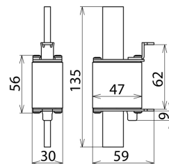
Maßbild VA NH1 280
