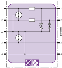
Prinzipschaltbild BXT ML2 BE S 12
