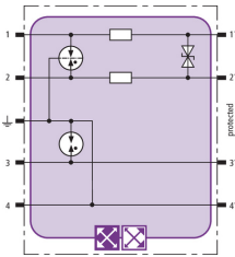
Prinzipschaltbild BXT ML2 BD S 5
