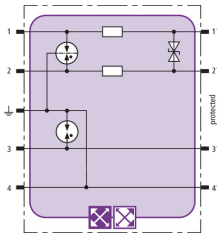
Prinzipschaltbild BXT ML2 BD S 48
