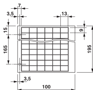
Maßzeichnung
