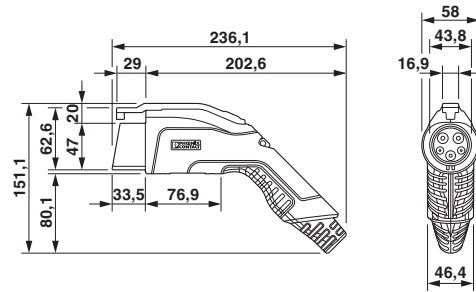
Maßzeichnung Fahrzeug-Ladestecker
