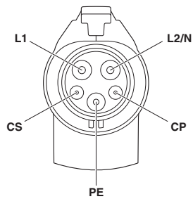
Pinbelegung Fahrzeug-Ladestecker
