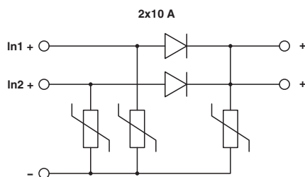
Blockschaltbild
