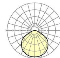
Lichttechnik freistrahlend-direkt freistrahlend SDGVL LED 7000 lm 840
