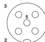
Polbild Buchse M12, 5-polig, A-kodiert, Ansicht Buchsen- und Polseite
