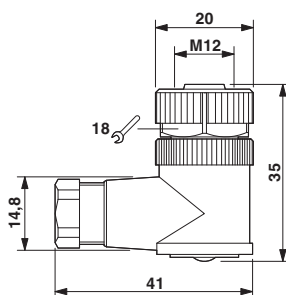
Maßzeichnung
