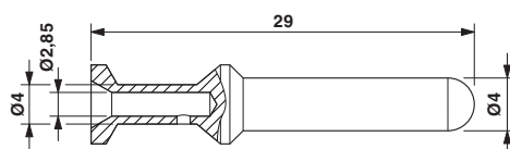
Maßzeichnung
