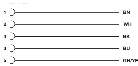
Kontaktbelegung der M12-Buchsen
