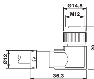
Maßzeichnung
