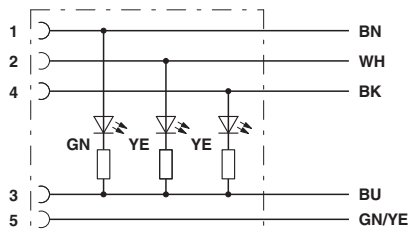
Schaltplan
