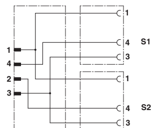
Schaltplan
