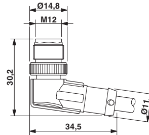
Maßzeichnung
