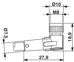
Maßzeichnung
