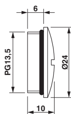
Maßzeichnung
