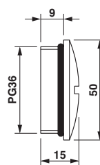
Maßzeichnung
