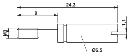
Maßzeichnung
