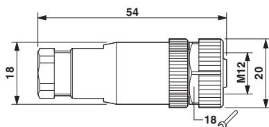
Buchse M12 x 1, gerade
