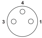
Polbild M8-Buchse, 3-polig
