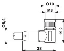
Buchse M8 x 1, gewinkelt, mit LED
