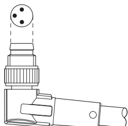
Schemazeichnung
