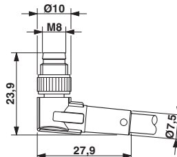
Maßzeichnung
