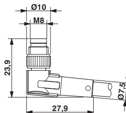
Maßzeichnung
