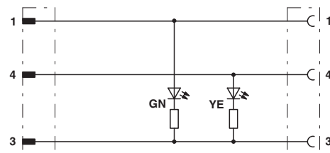
Kontaktbelegung der M8-Stecker / M12-Buchse
